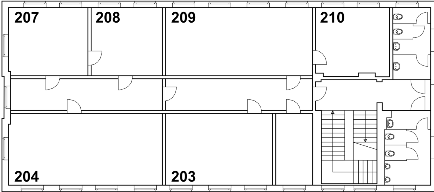
2. Obergeschoss
